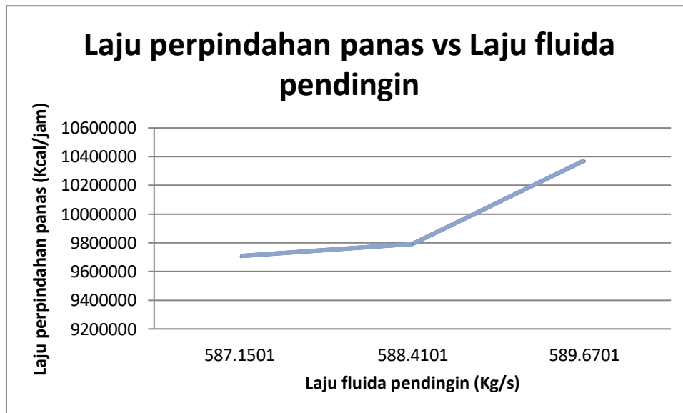
Gambar 3. Grafik laju perpindahan panas VS laju fluida pendingin
