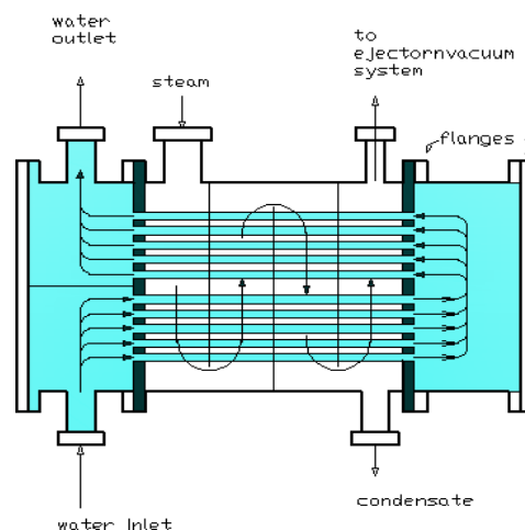
Gambar 1. mekanisme kerja daripada kondensor
