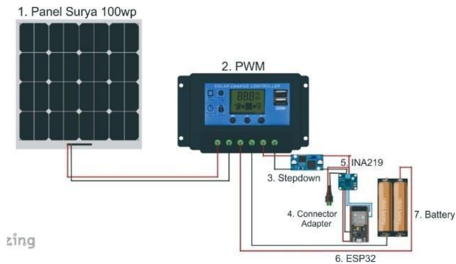
Gambar 2. Desain skematik
