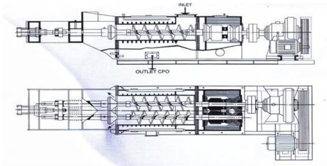
Gambar 1. Keterpasangan screw press dan tekanan hidrolik
