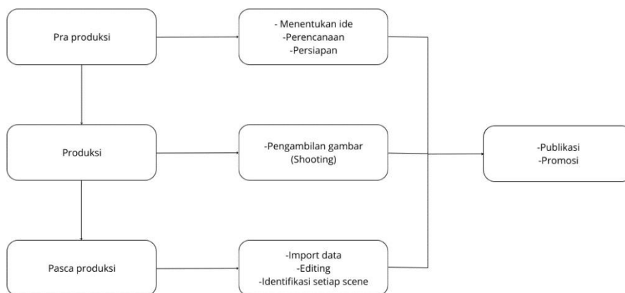
Gambar 1 Tahapan Penelitian
