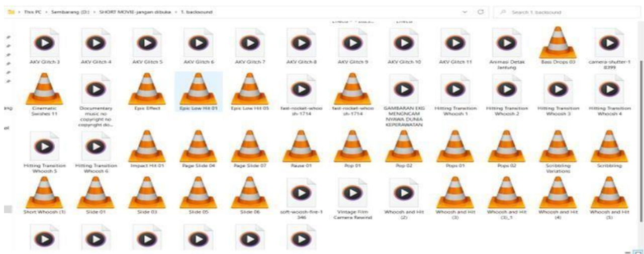
Gambar 3 Pemilihan audio
