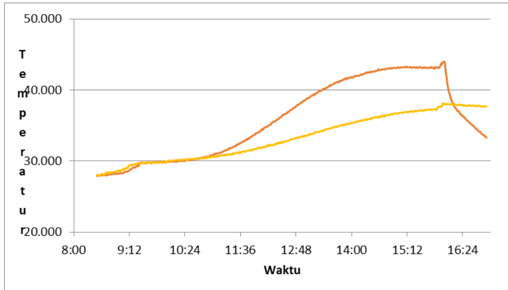
Gambar 3. Grafik Temperatur Pelat Absorber dan Air Vs Waktu
