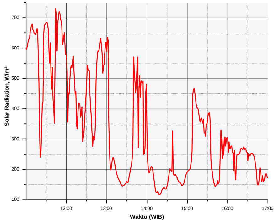
Gambar 5. Grafik Intensitas Matahari Vs Waktu
