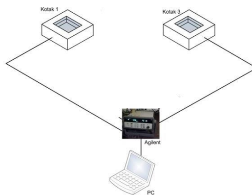
Gambar 2. Skema Pengambilan Data Pemanas Air Tenaga Surya
