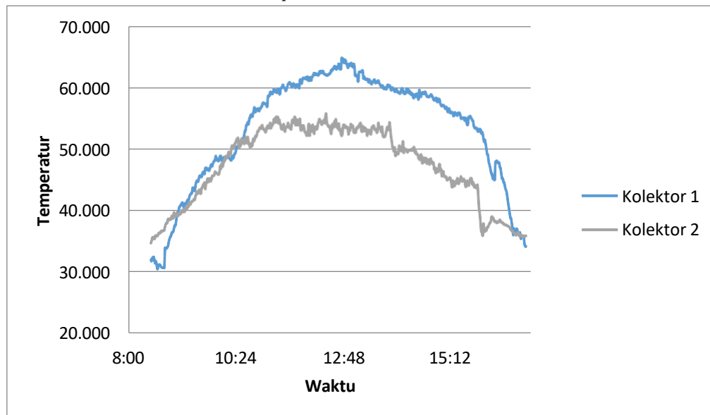
Gambar 4. Grafik Temperatur Pelat Absorber dan Air Vs Waktu
