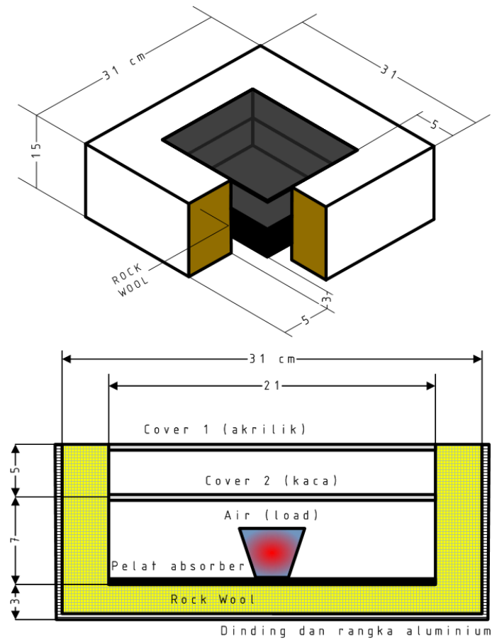
Gambar 1. Skema Kotak Kolektor
