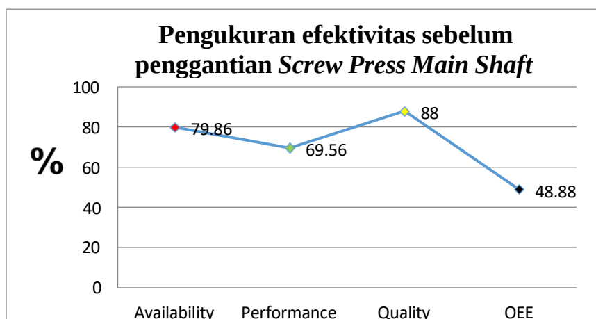
Gambar 3. Grafik pengukuran efektivitas kinerja mesin Expeller Pressing sebelum penggantian Screw Press Main Shaft .
